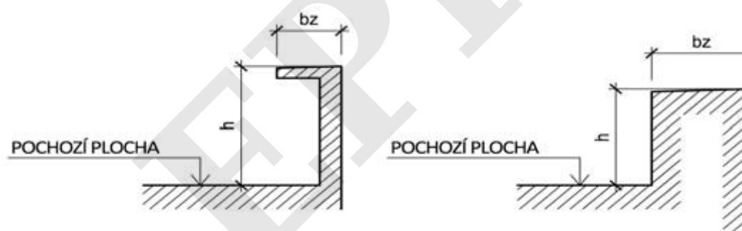
Obrázek 6: Příklady zvětšené šířky zábradlí
