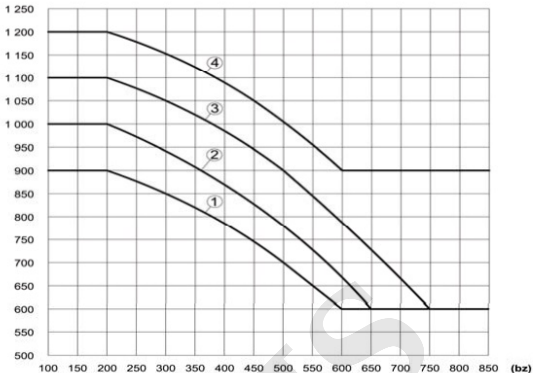
Nejmenší dovolené výšky zábradlí (mm): 1 - snížená, 2 - základní, 3 - zvýšená, 4 - zvláštní Obrázek 7: Diagram výšky a šířky zábradlí
